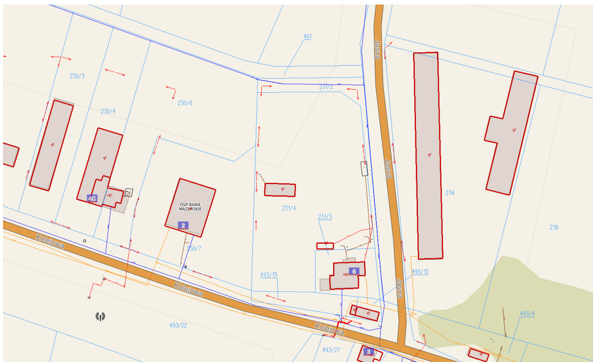
Rysunek 3. Dostępne sieci energetyczne i wodociągowe
